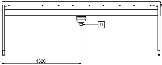
Zij aanzicht
