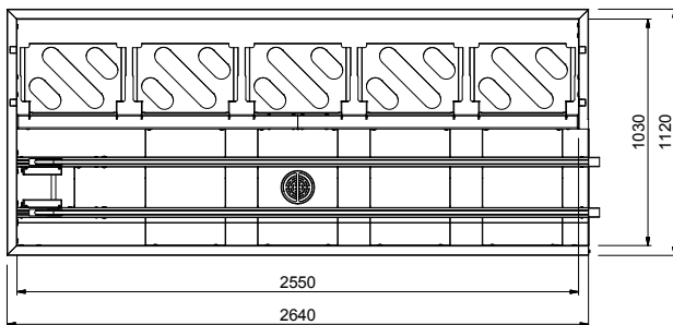
Boven aanzicht
